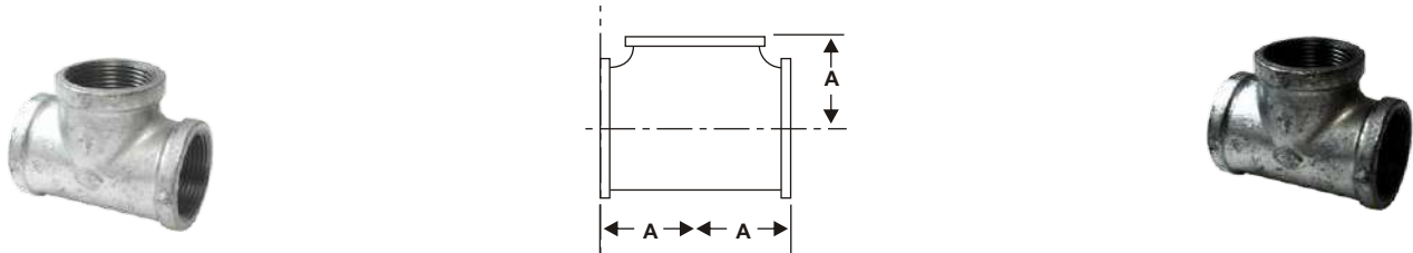
Fig 130 Tee
