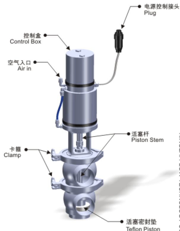
316Lss 气动活塞阀 外观指示图 316Lss Air Actuated Piston Valves Exterior Description
